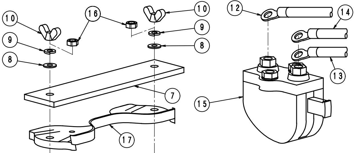
FIG-7バッテリー系
