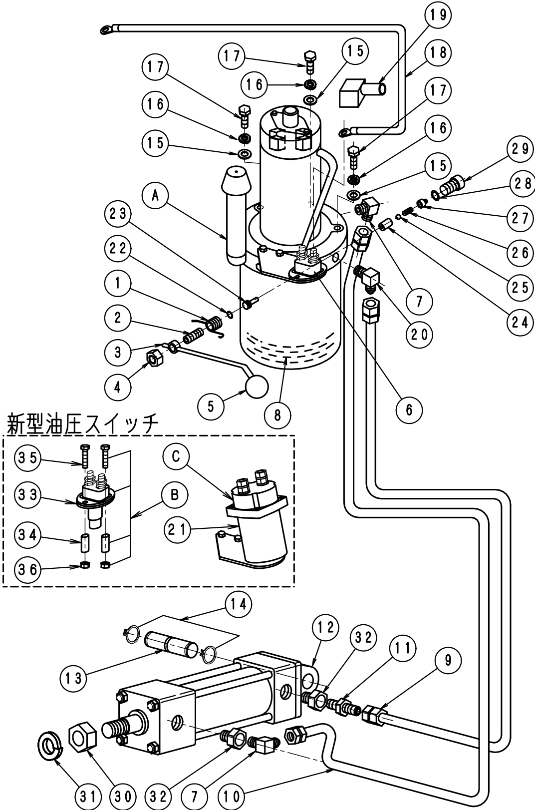
FIG-9油圧系
