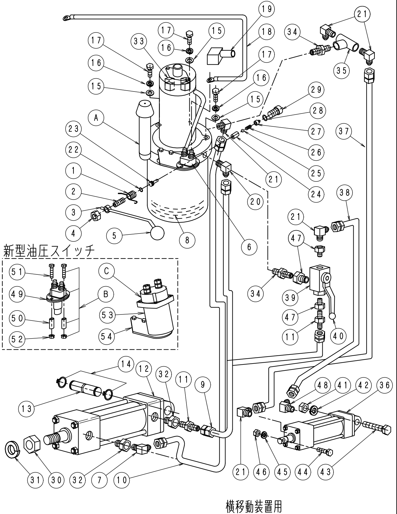
FIG-9油圧系
