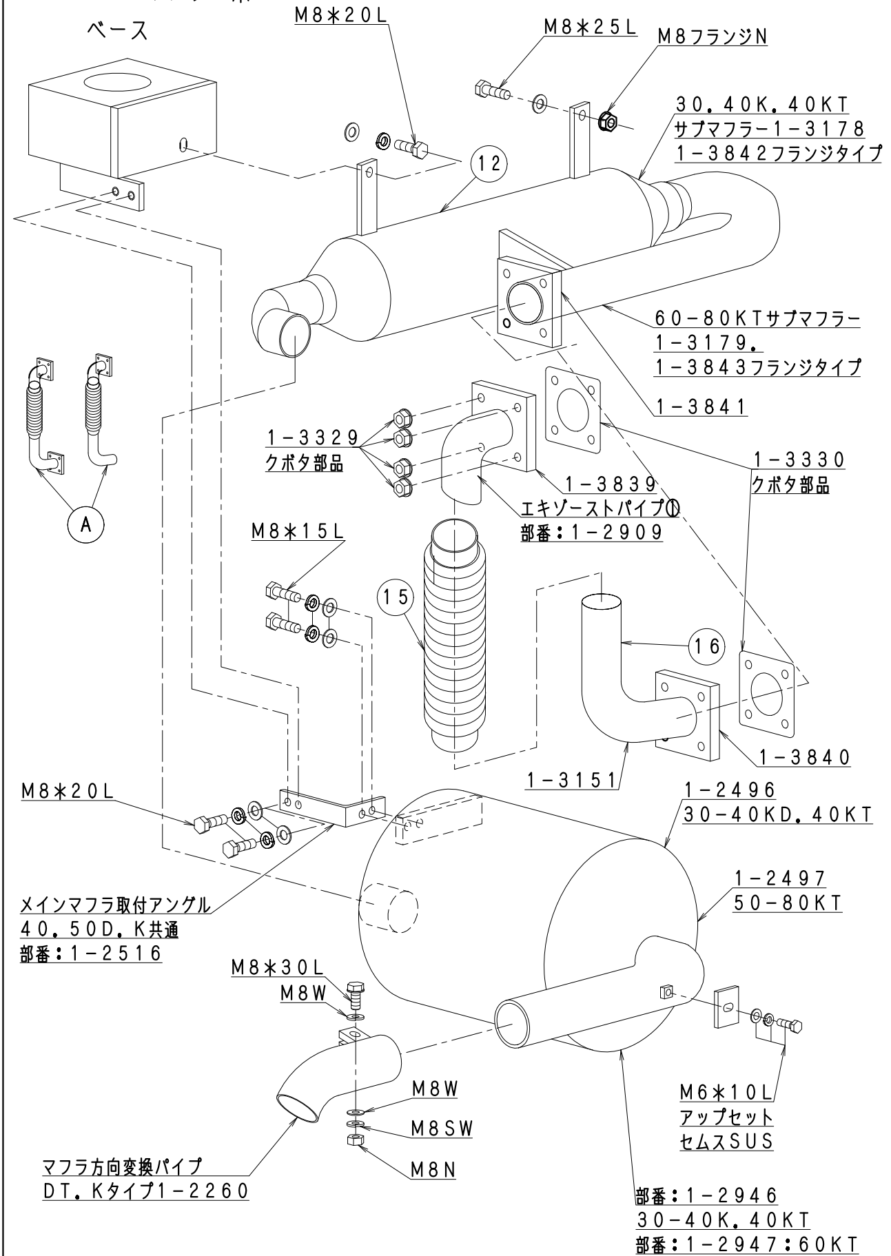
FIG-13マフラー系
