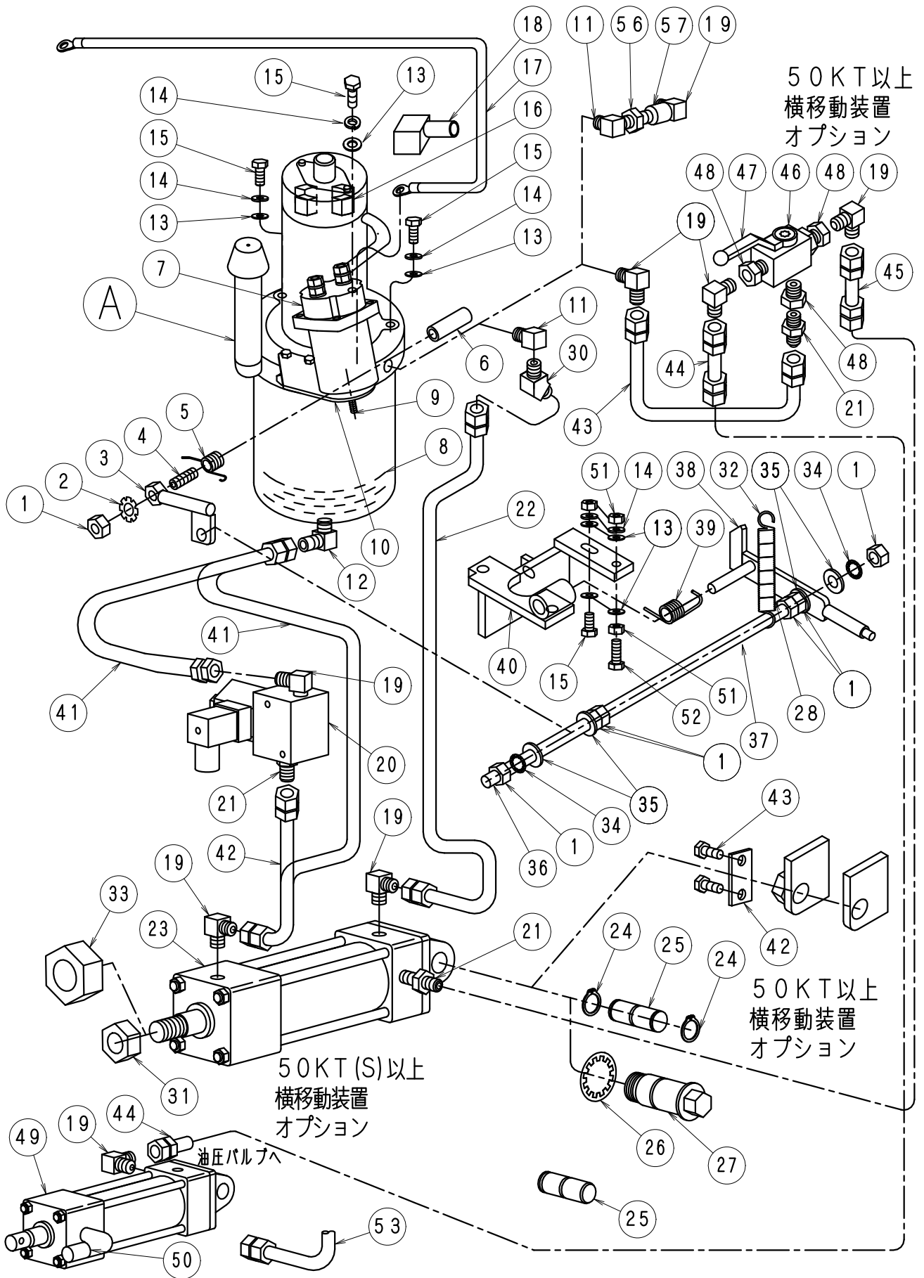
FIG-9 油圧系
