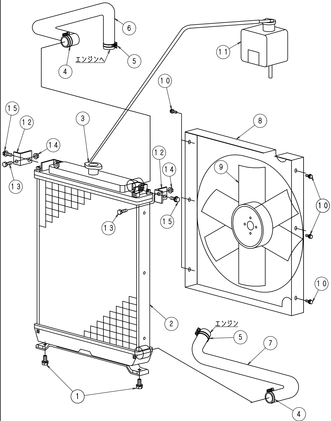
FIG-14 冷却系
