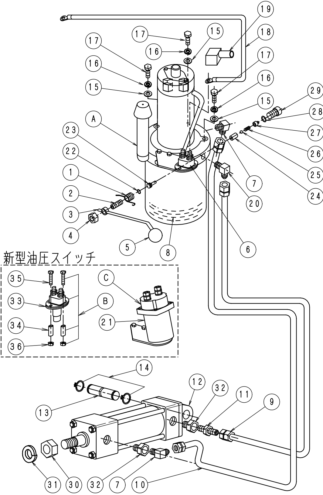
FIG-9油圧系
