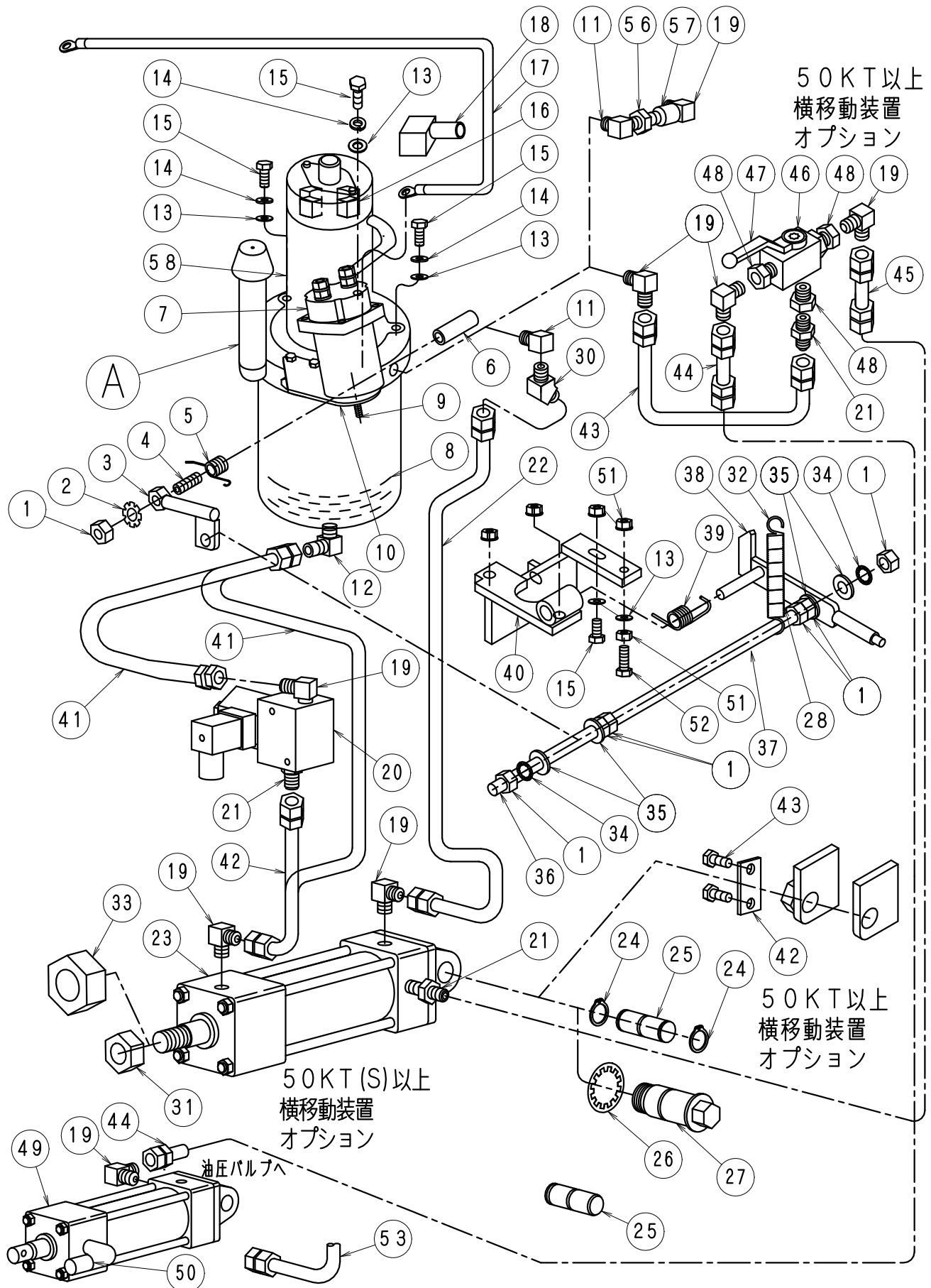
FIG-9 油圧系
