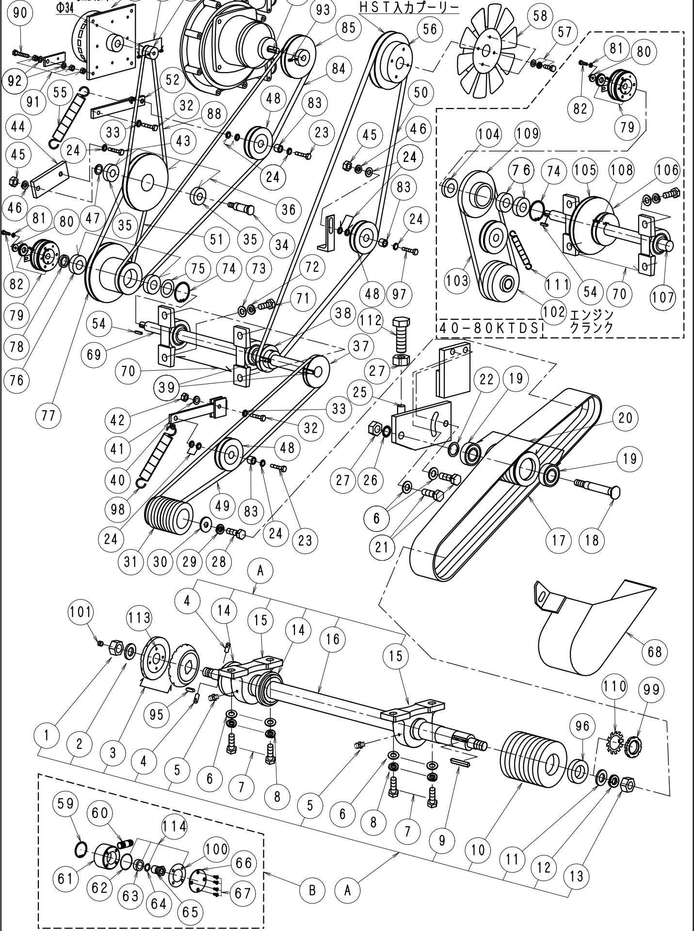
FIG-1 駆動系
