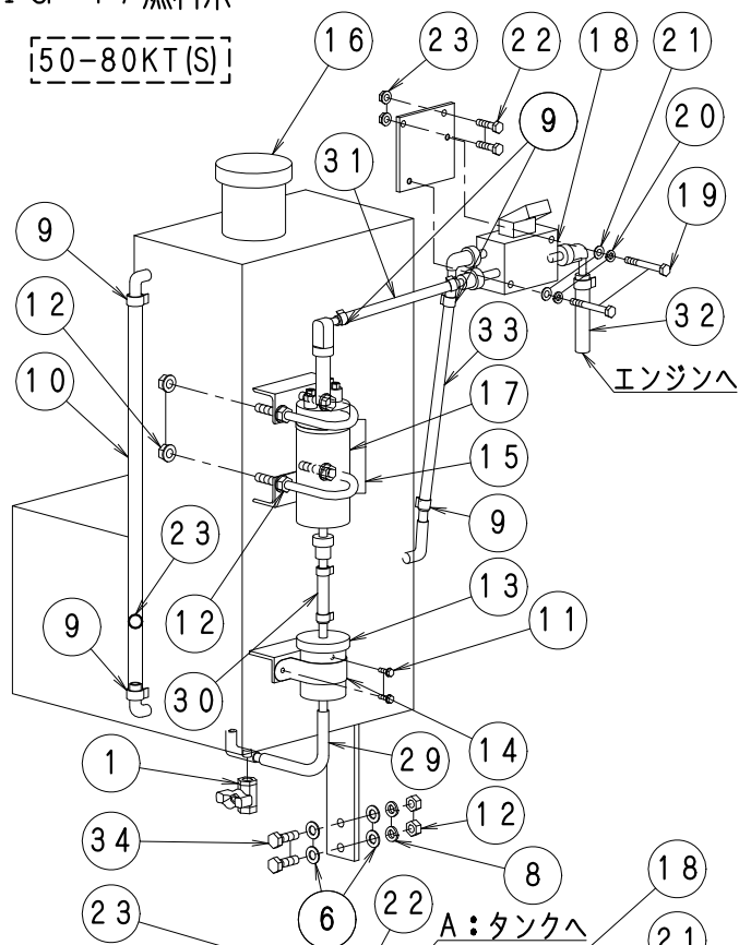
FIG-17 燃料系
