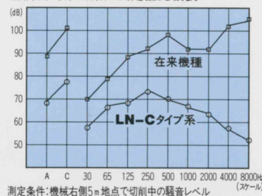
■防音対策効果/測定値比較表
