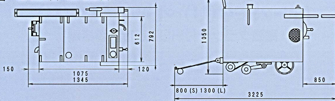
寸法図 LN-25EO(U)~LN-40EO(U)
