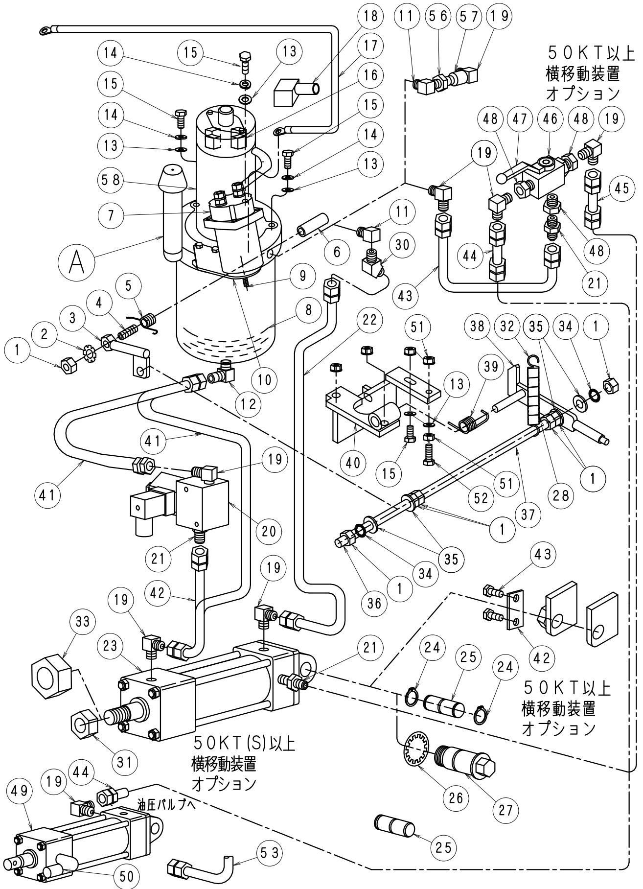
FIG-9 油圧系
