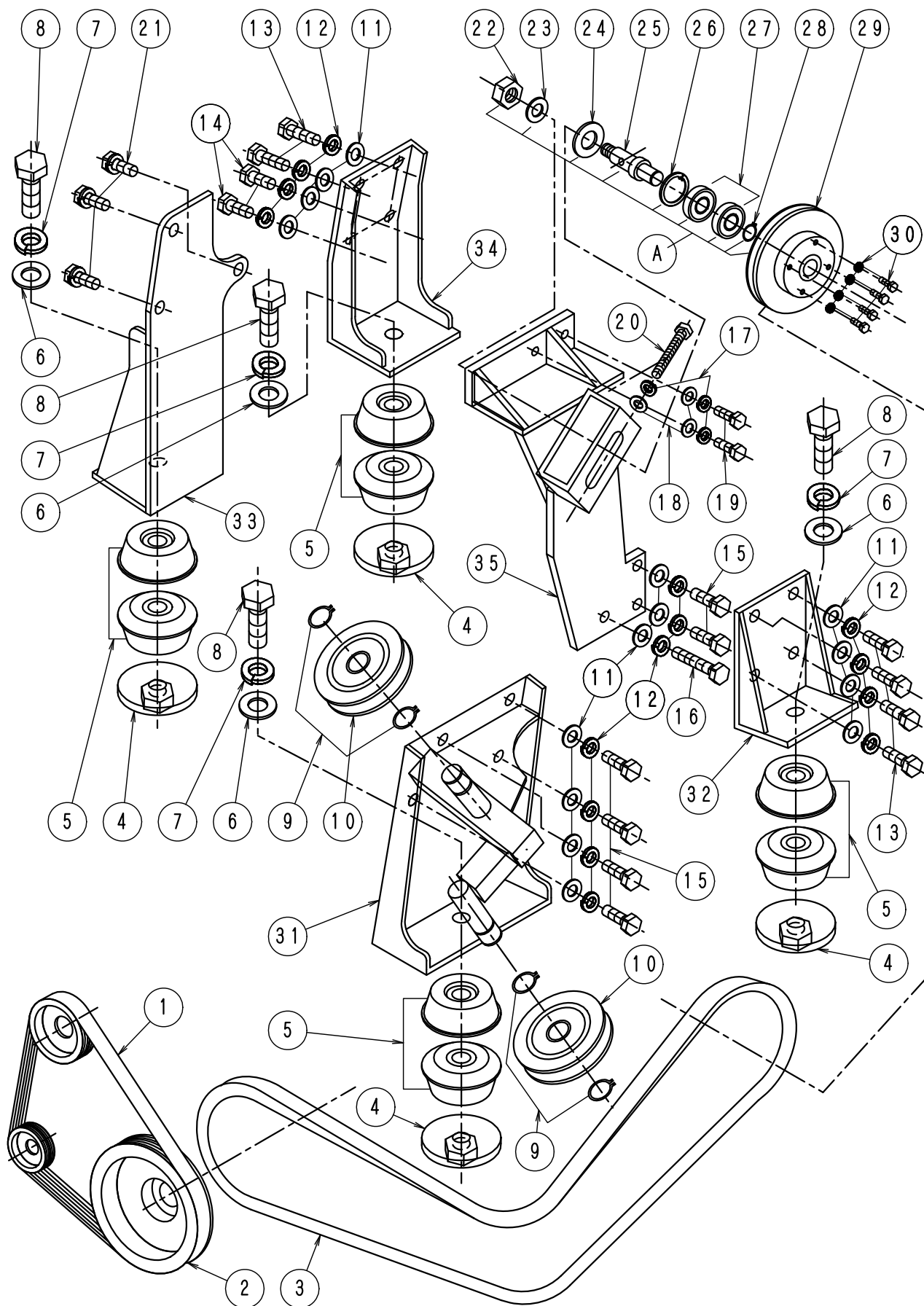
FIG-10 ファンプーリー系
