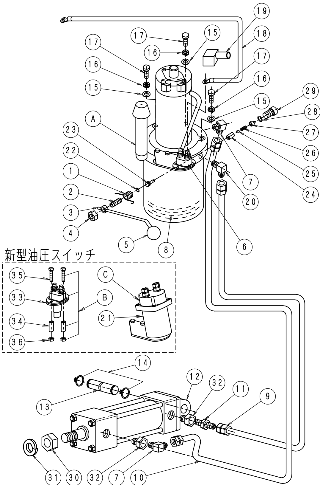
FIG-9 油圧系
