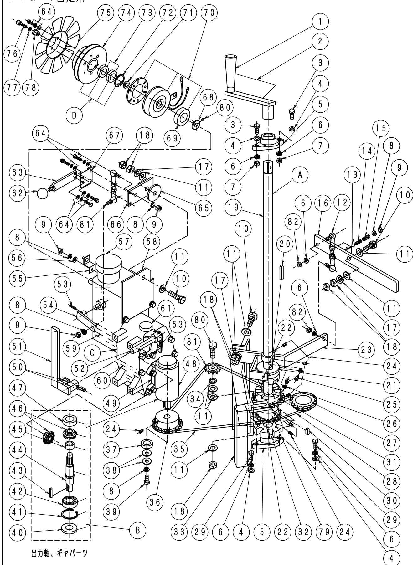
FIG-4 自走系
