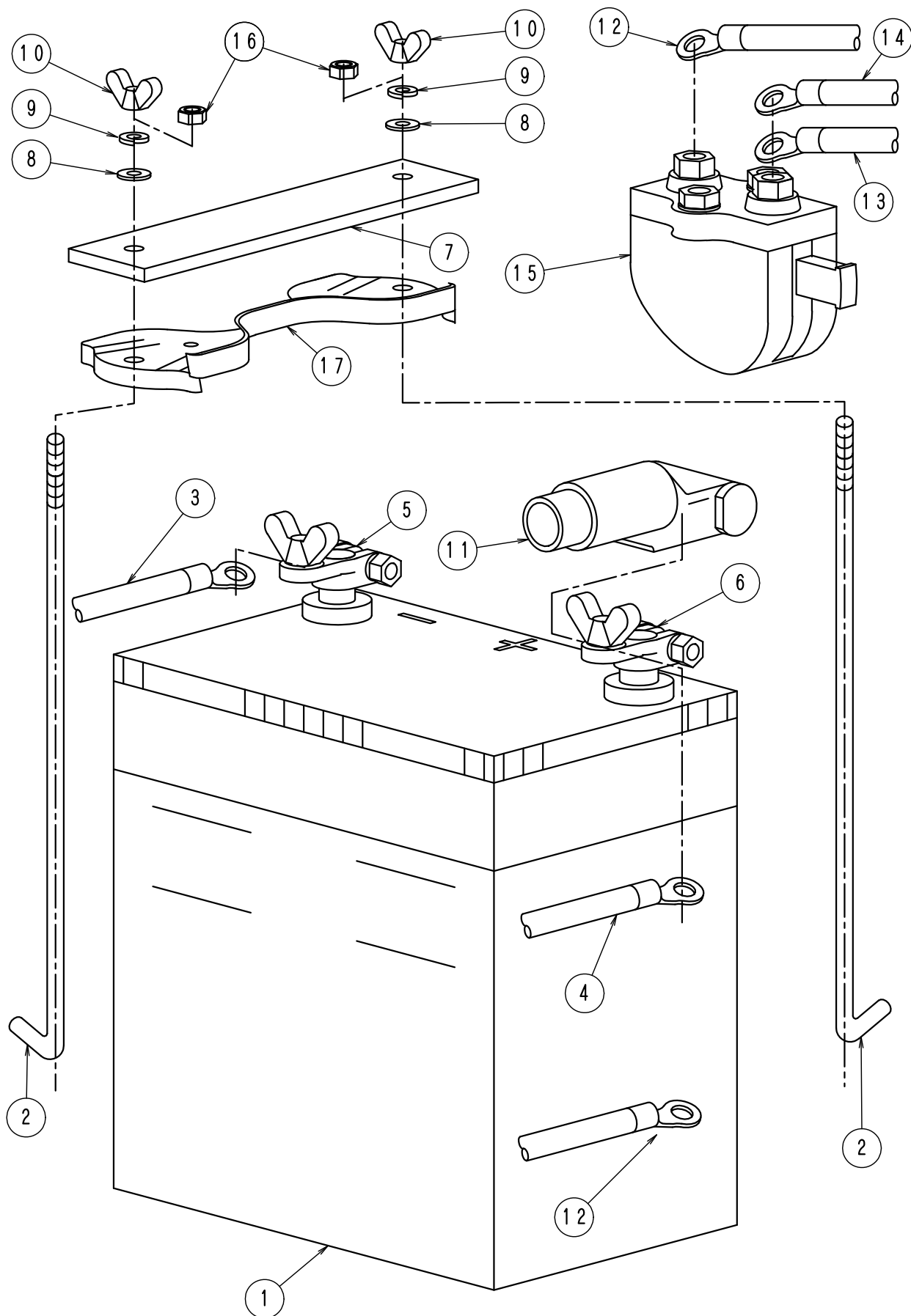
FIG-7バッテリー系
