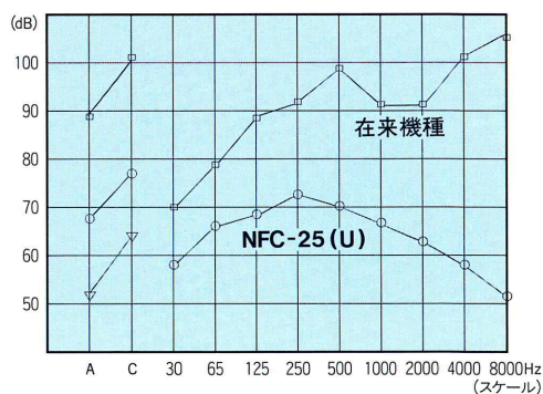
■ 防音対策効果／測定値比較表
