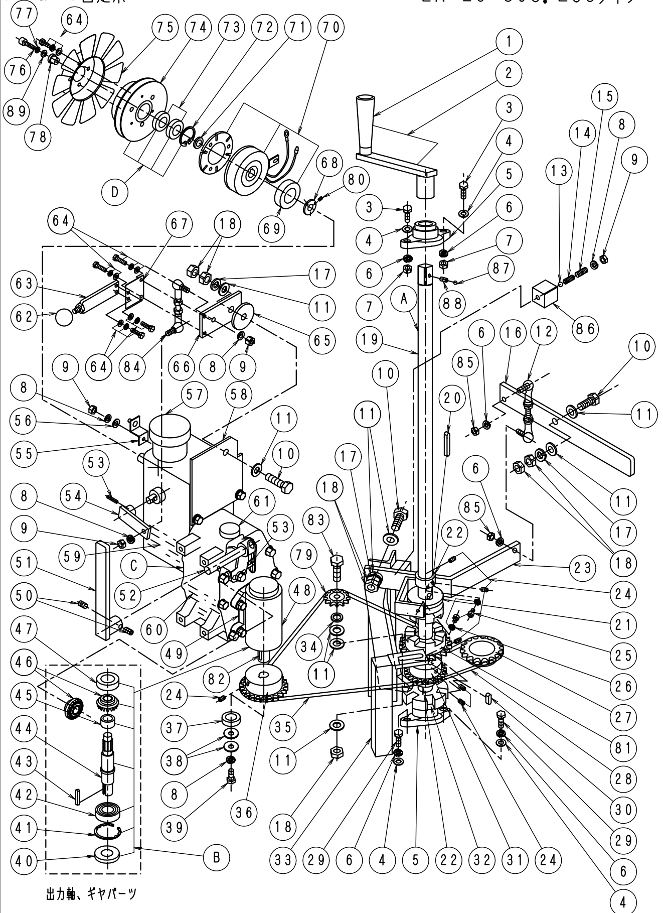
FIG-4 自走系
