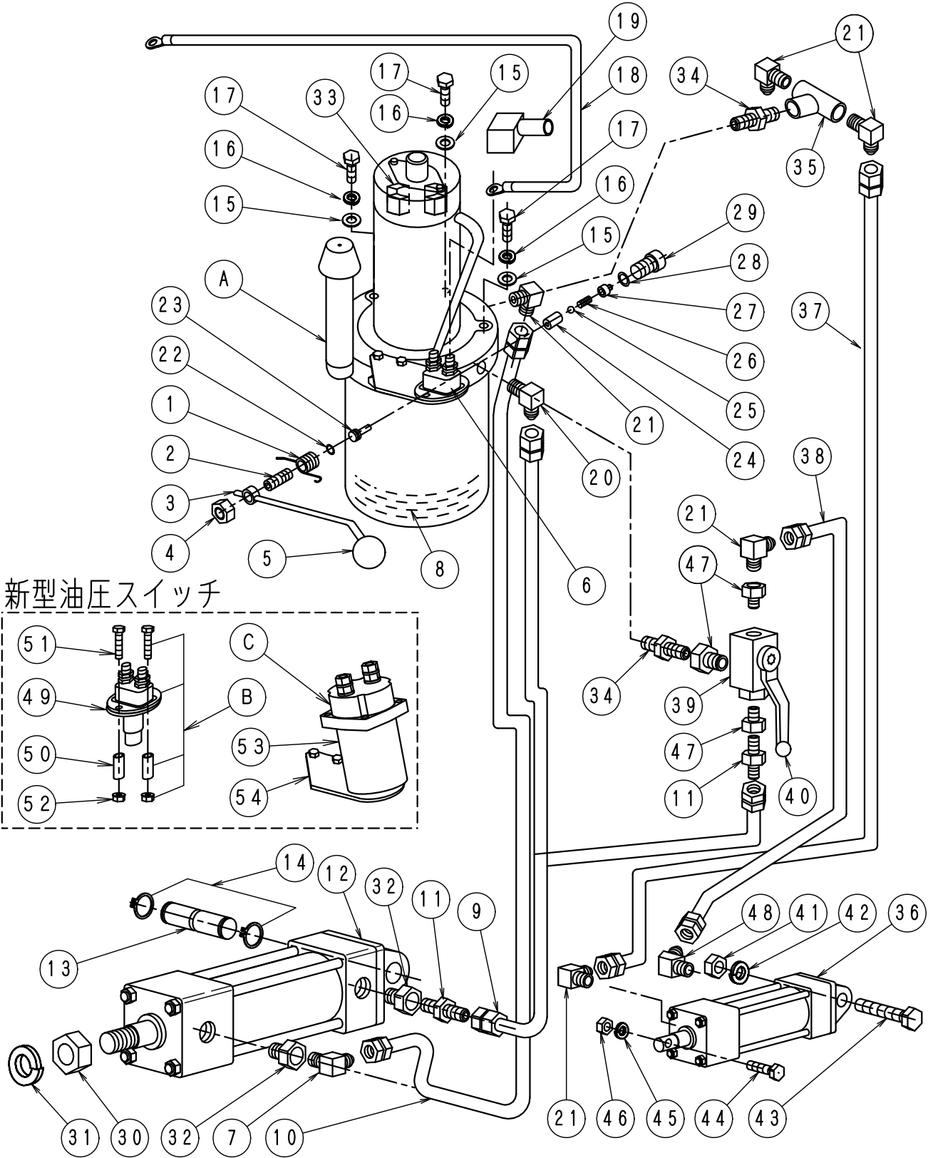
FIG-9油圧系
