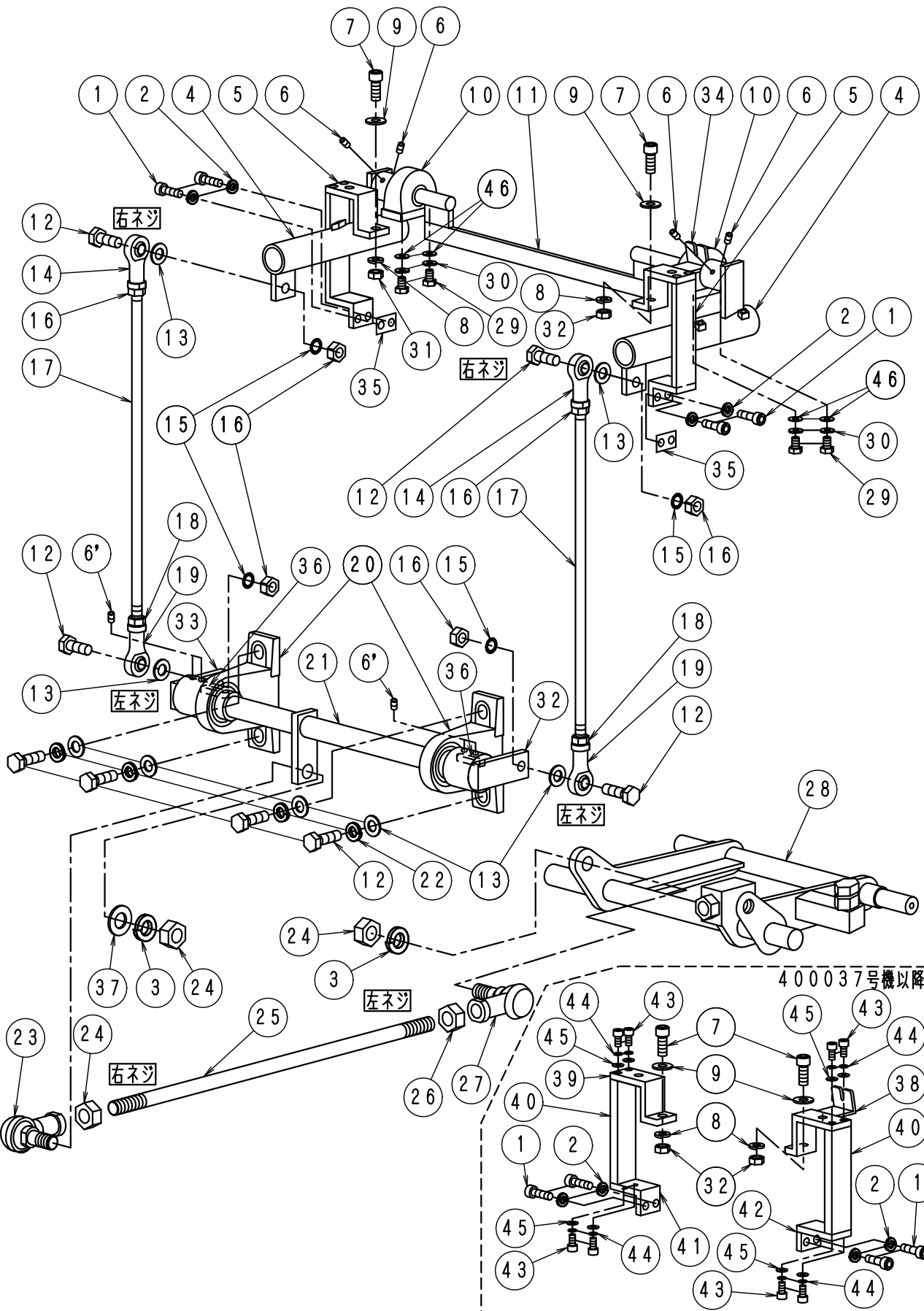
FIG-12 可変操作系
