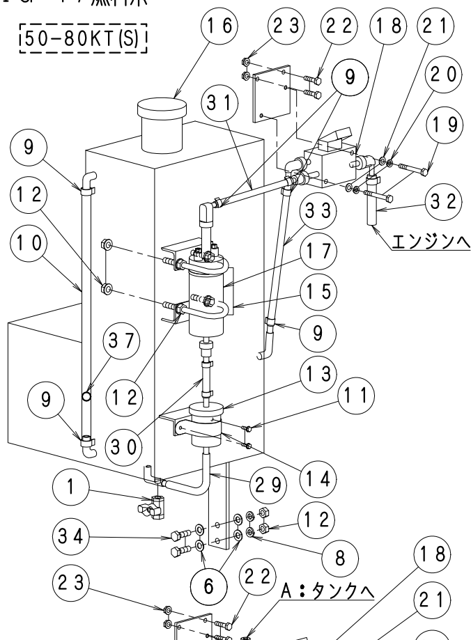
FIG-17 燃料系
