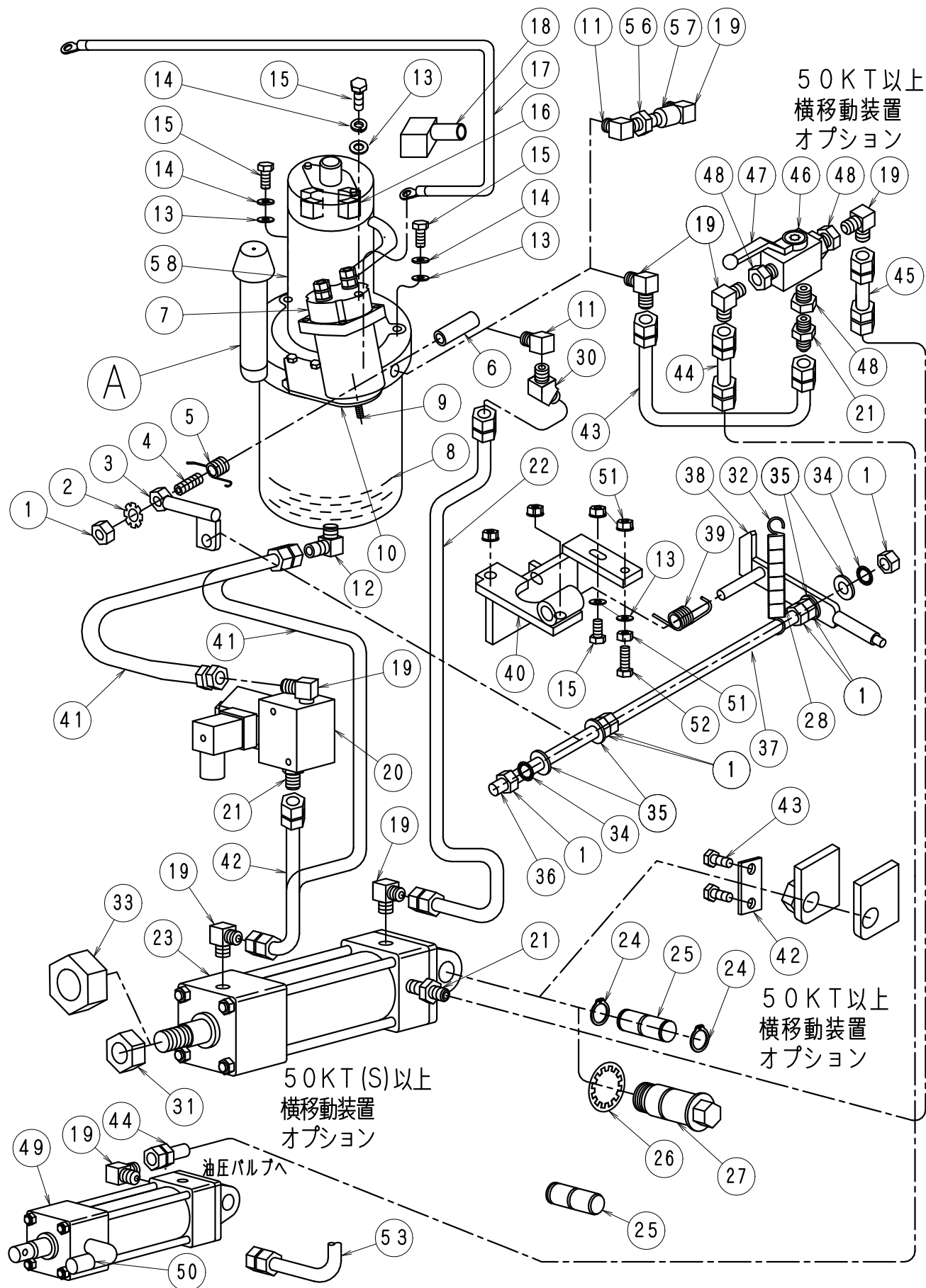
FIG-9 油圧系
