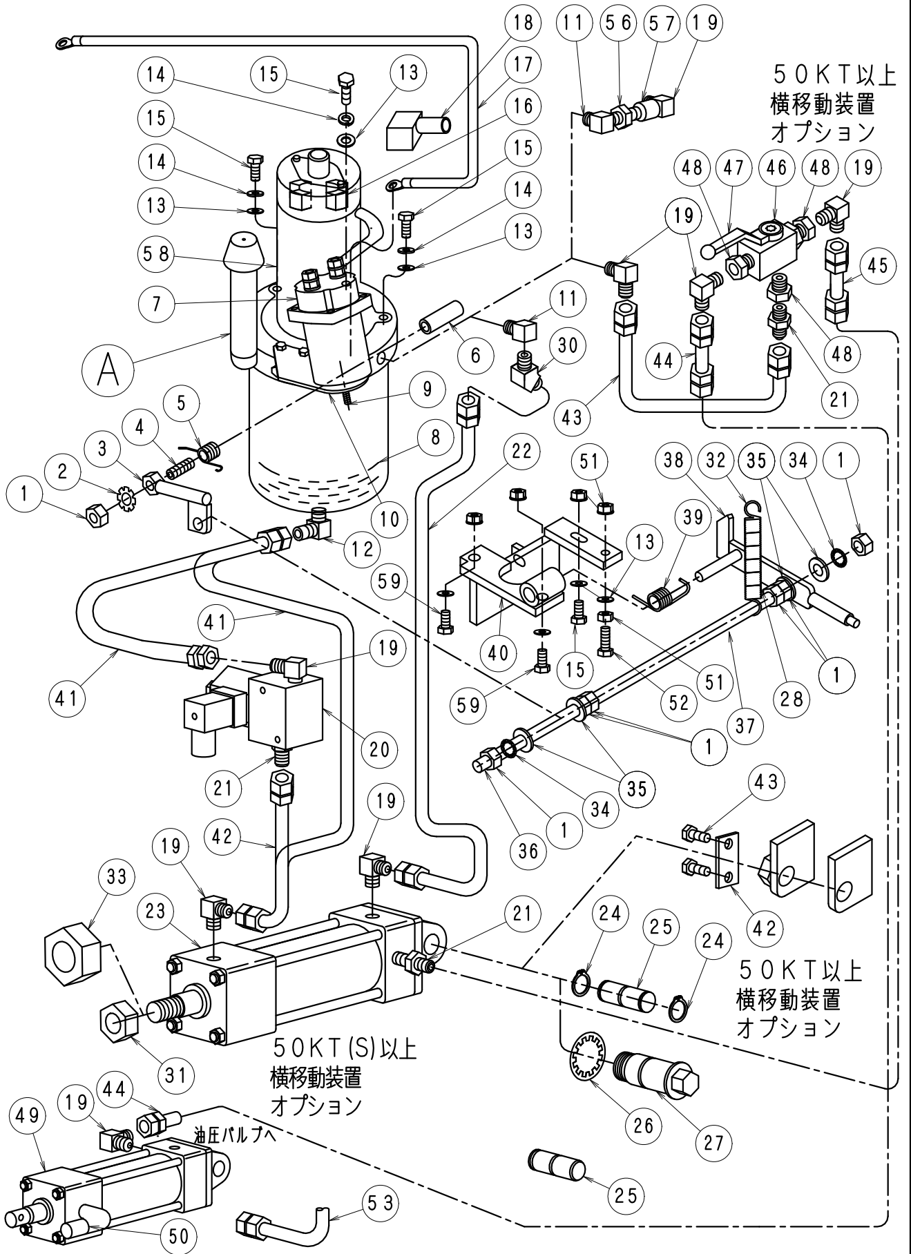
FIG-9 油圧系
