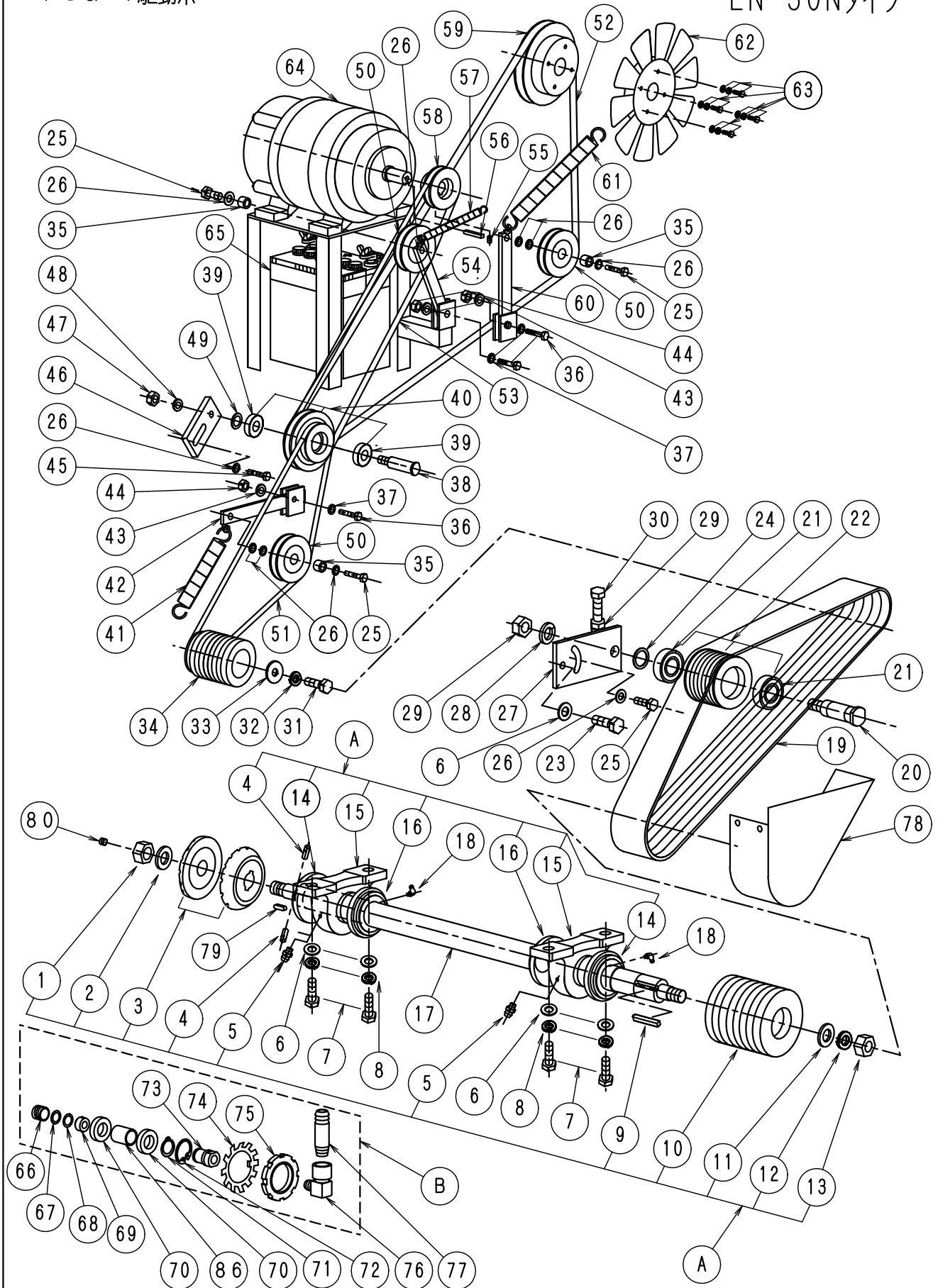
FIG-1 駆動系
